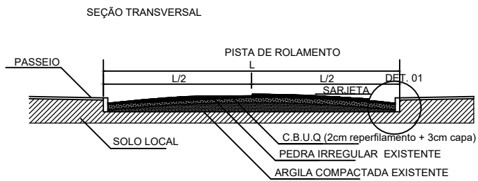
SEÇÃO TRANSVERSAL TÍPICA Esc Indet.
