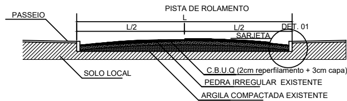
SEÇÃO TRANSVERSAL TÍPICA Esc Indet.
