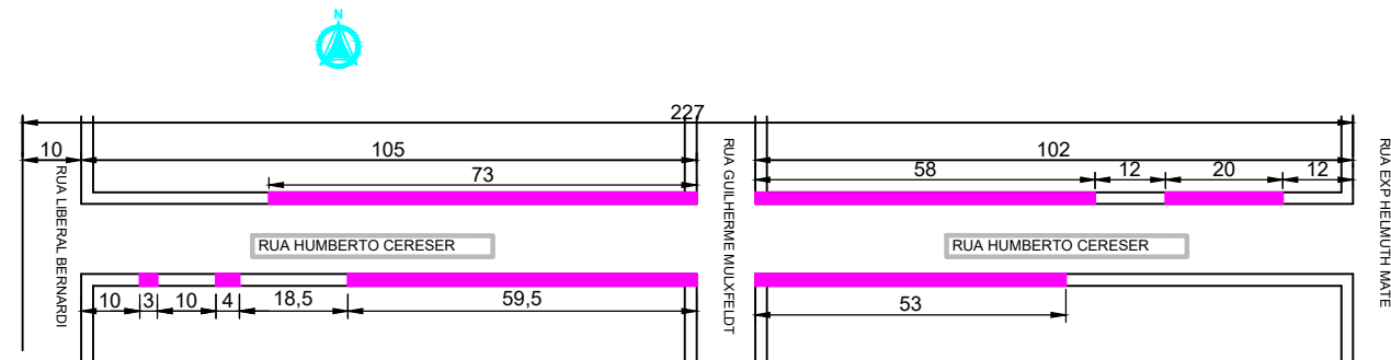
PLANTA BAIXA SUBSTITUIÇÃO DE MEIO FIO
