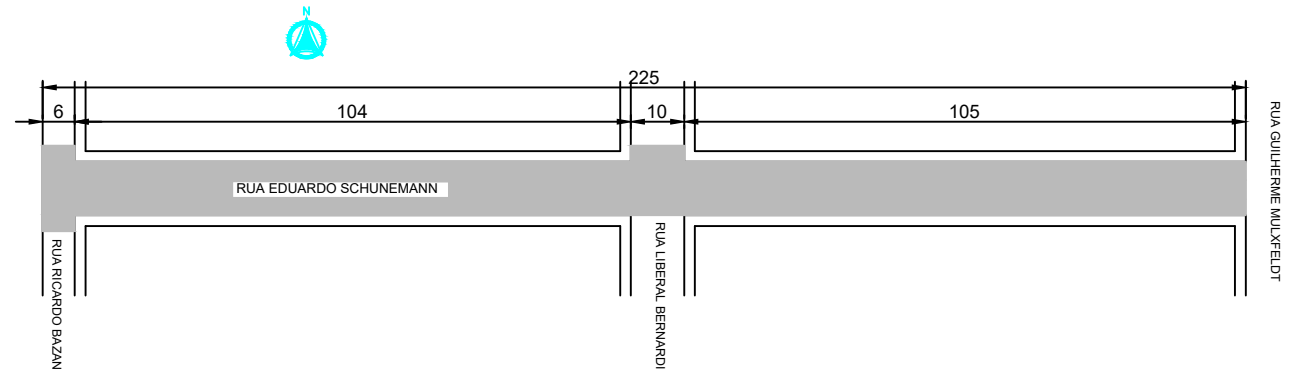
PLANTA BAIXA PAVIMENTAÇÃO ASFÁLTICA
