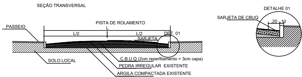
SEÇÃO TRANSVERSAL TÍPICA Esc. Indet.
