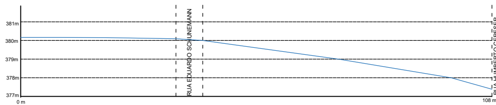
PERFIL LONGITUDINAL
