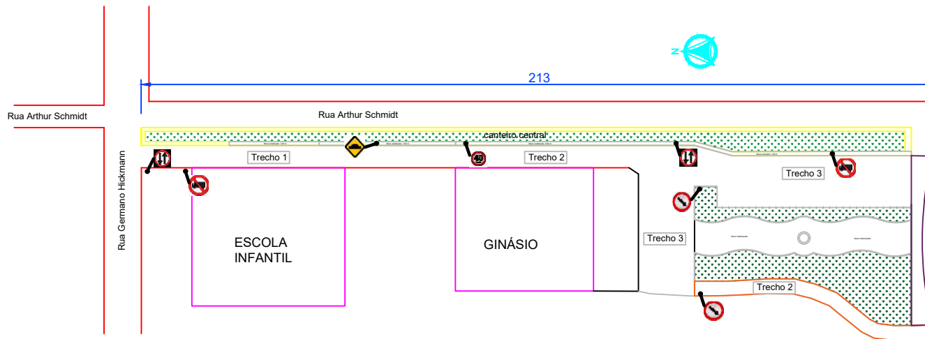
PLANTA BAIXA SINALIZAÇÃO
