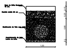
CORTE AB ESCALA IND.
