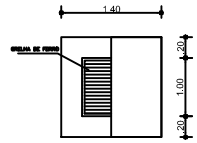
CAIXA DE CAPTAÇÃO PLANTA BAIXA ESCALA IND.
