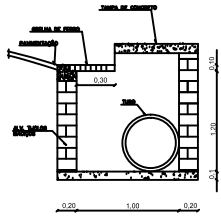
CORTE AB ESCALA IND.
