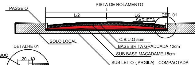
SEÇÃO TRANSVERSAL TÍPICA Esc Indet.
