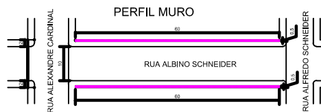
PERFIL MURO
