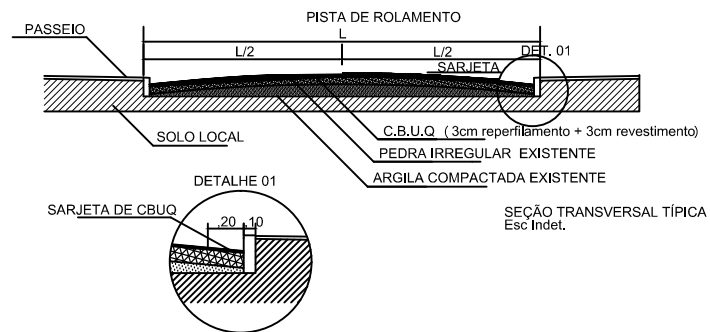
SEÇÃO TRANSVERSAL
