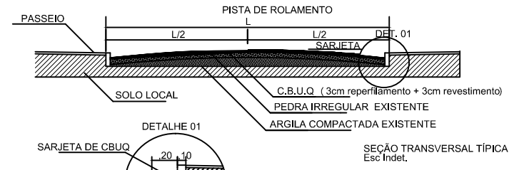
SEÇÃO TRANSVERSAL
